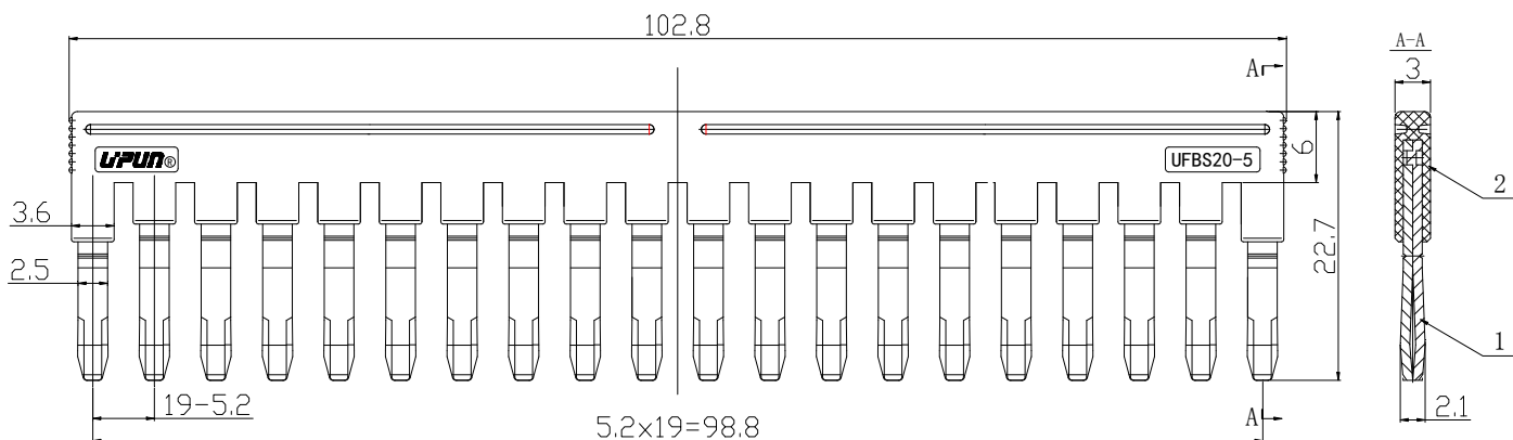
公差表
