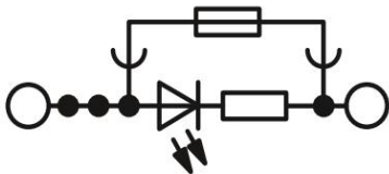
电路图
