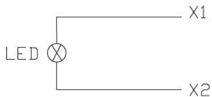
接线图
