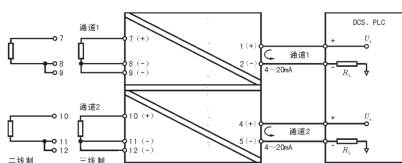
接线图
