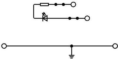
电路图
